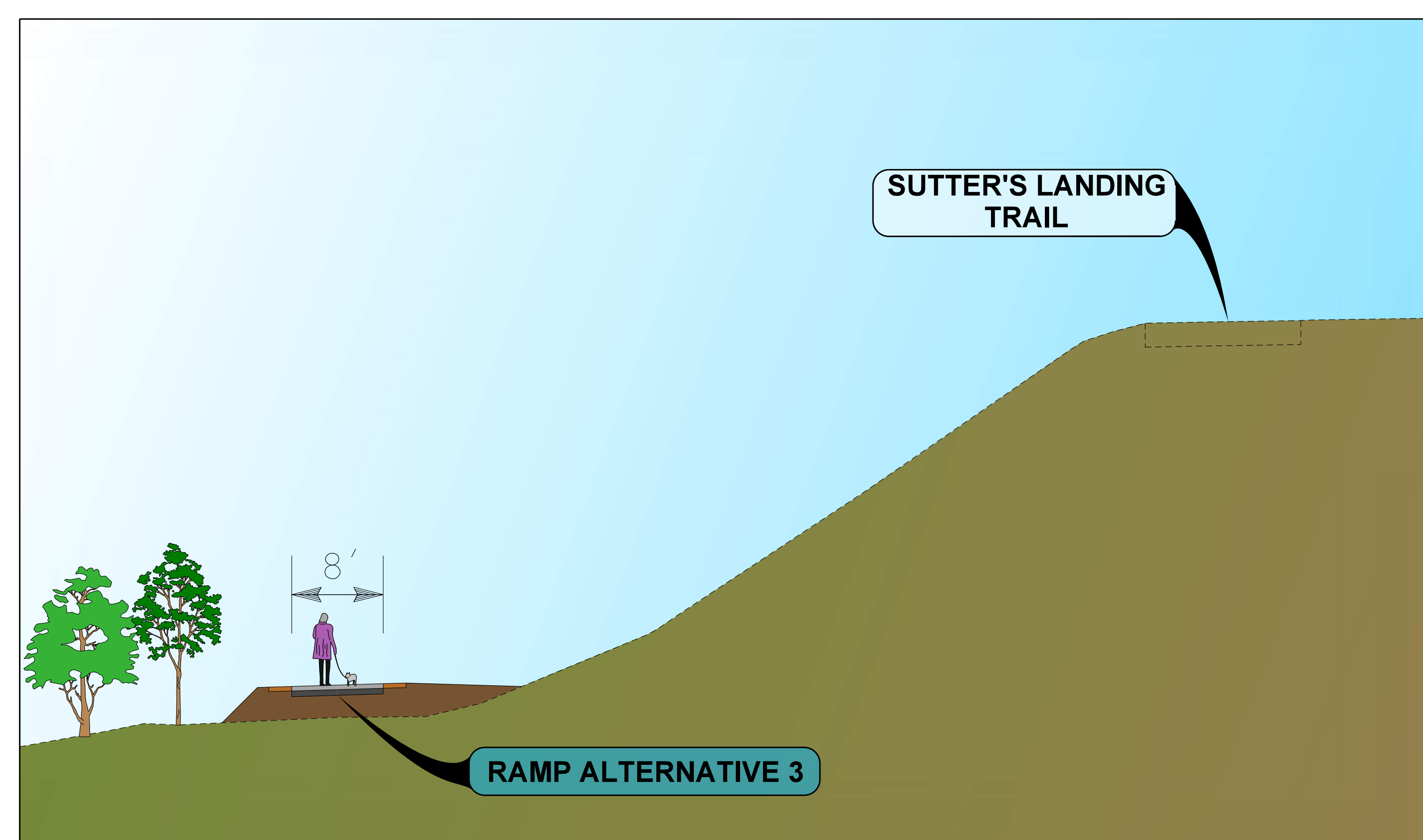
SECTION A-A
